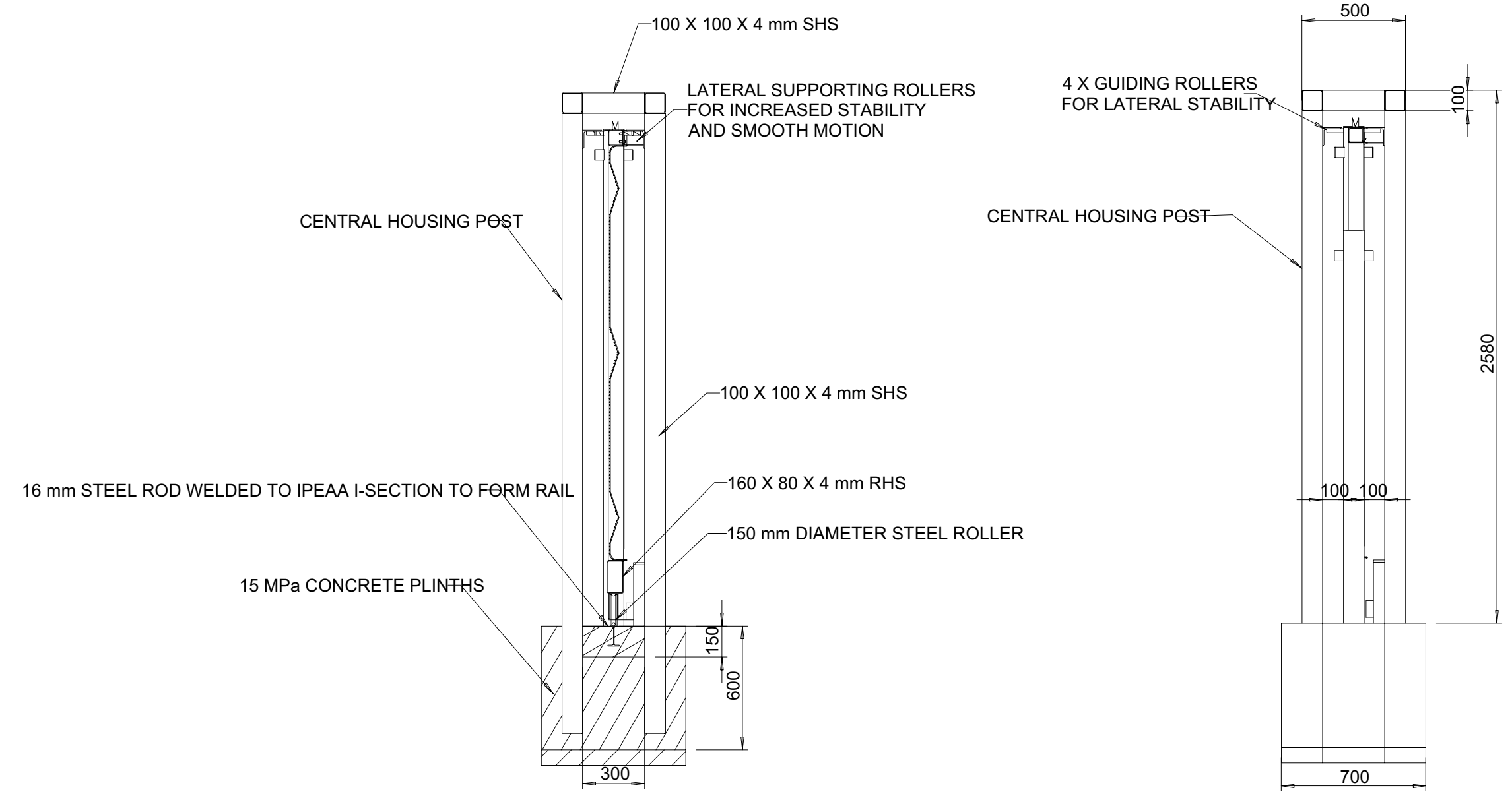
SECTION D 1:25
