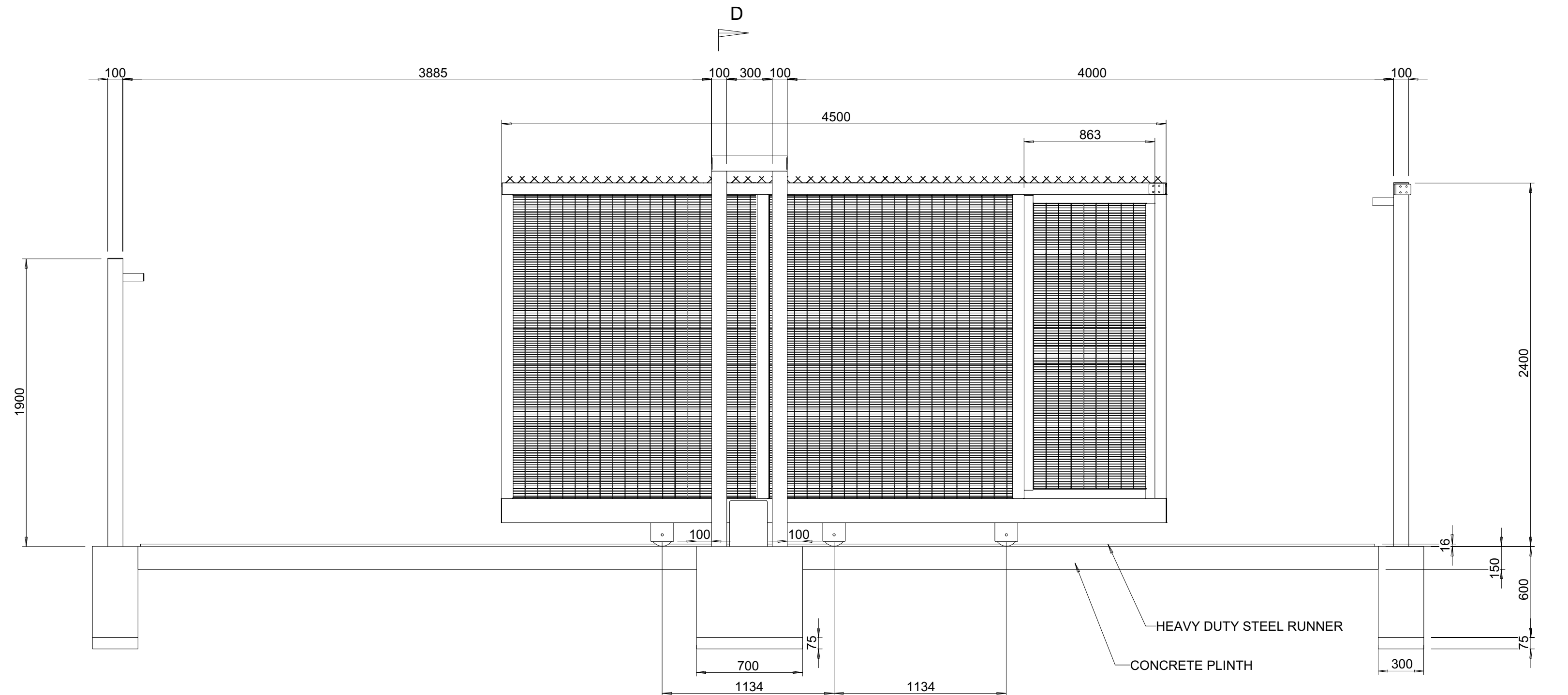
ELEVATION 1:25
