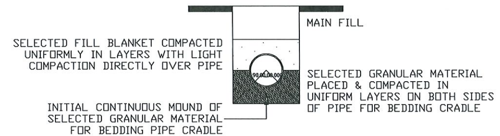
RIGID PIPE ON CLASS B BEDDING N.T.S
