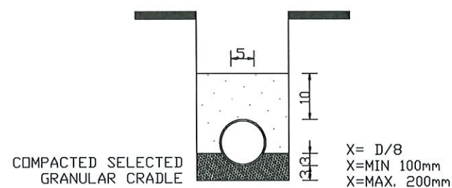
RIGID PIPE ON CLASS C BEDDING N.T.S
