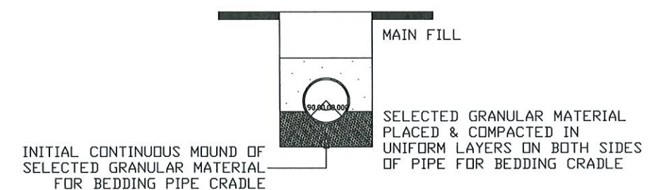
RIGID PIPE ON CLASS B BEDDING N.T.S
