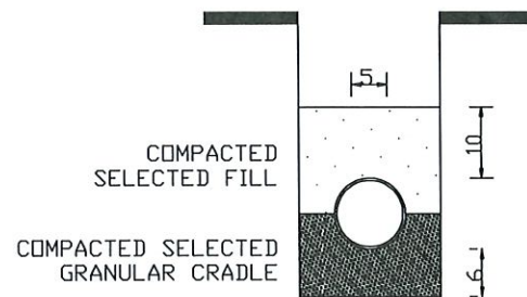
RIGID PIPE ON CLASS B BEDDING N.T.S
