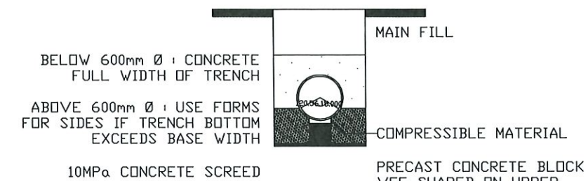
RIGID PIPE ON CLASS A BEDDING N.T.S
