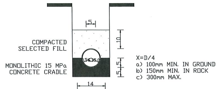
RIGID PIPE ON CLASS A BEDDING N.T.S
